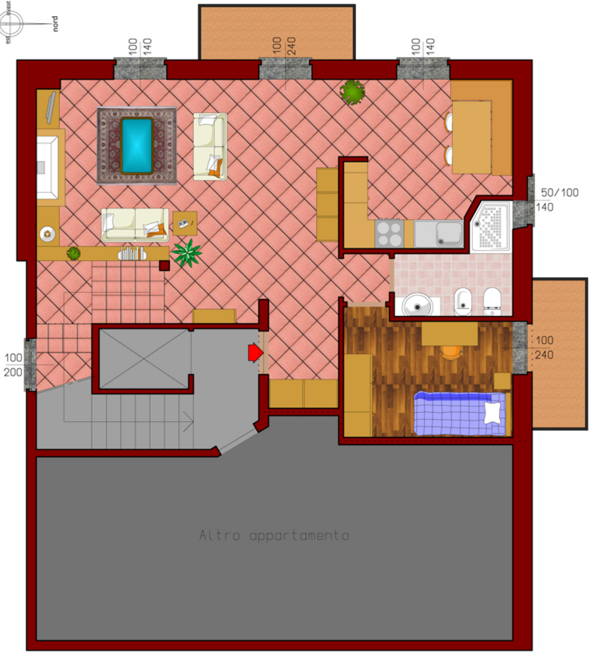
PIANTA PIANO SECONDO
